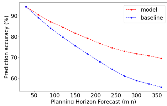
(d) EWR Model accuracy Vs Baseline
